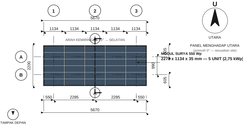
TAMPAK ATAS SKALA 1 : 100
